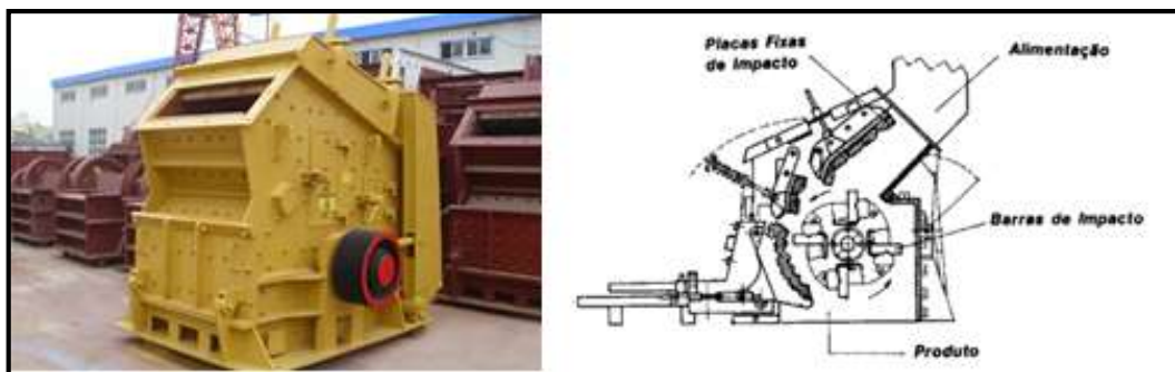
Figura 35. Exemplo e esquema de britador de impacto
