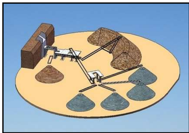
Figura 33. Esquema de URCC, com britagem e separação por tipo de resíduos e granulometria.
