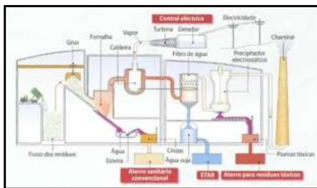
Figura 31. Funcionamento de uma central de tratamento térmico
