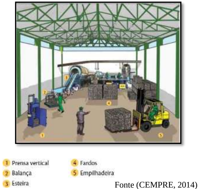
Figura 29. Layout interno de um galpão de triagem
